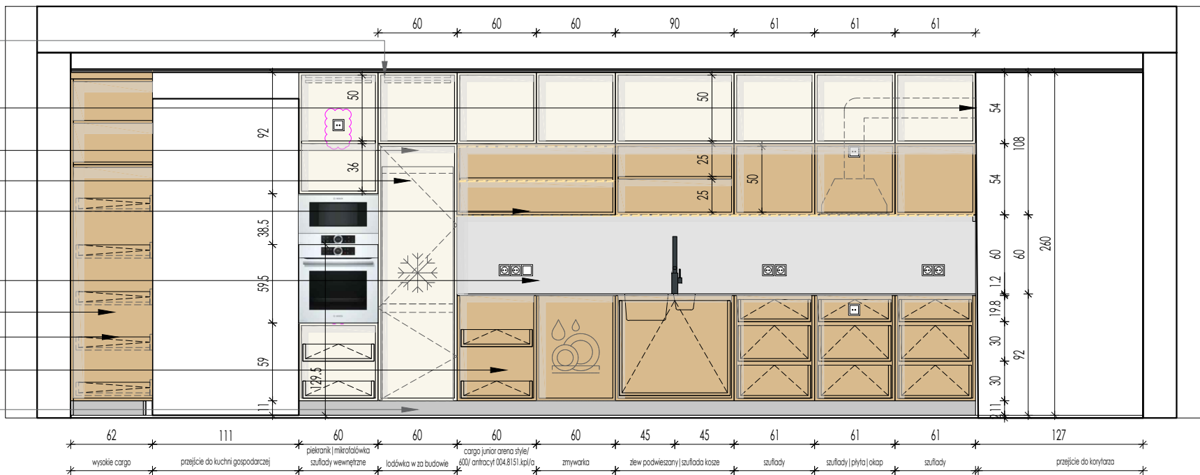
KUCHNIE WIDOK A-A SZAFKI OTWARTE
