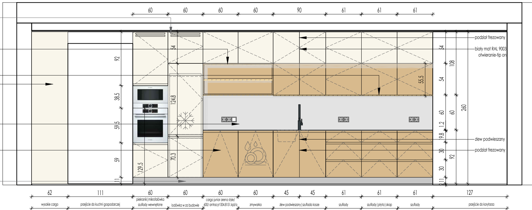
KUCHNIE WIDOK A-A
