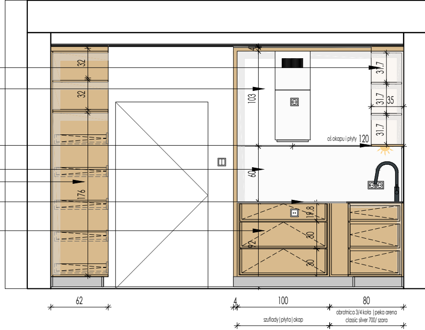
KUCHNIE WIDOK E-E
