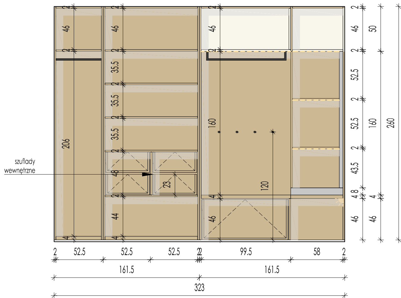
GARDEROBA PRZY HOLU-WIDOK B-B| OTWARTA
