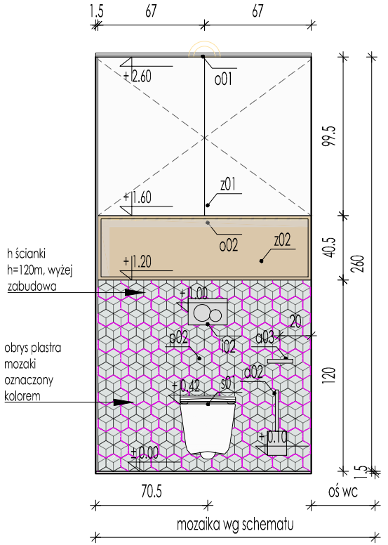
WIDOK B-B
