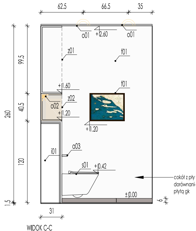
WIDOK C-C
