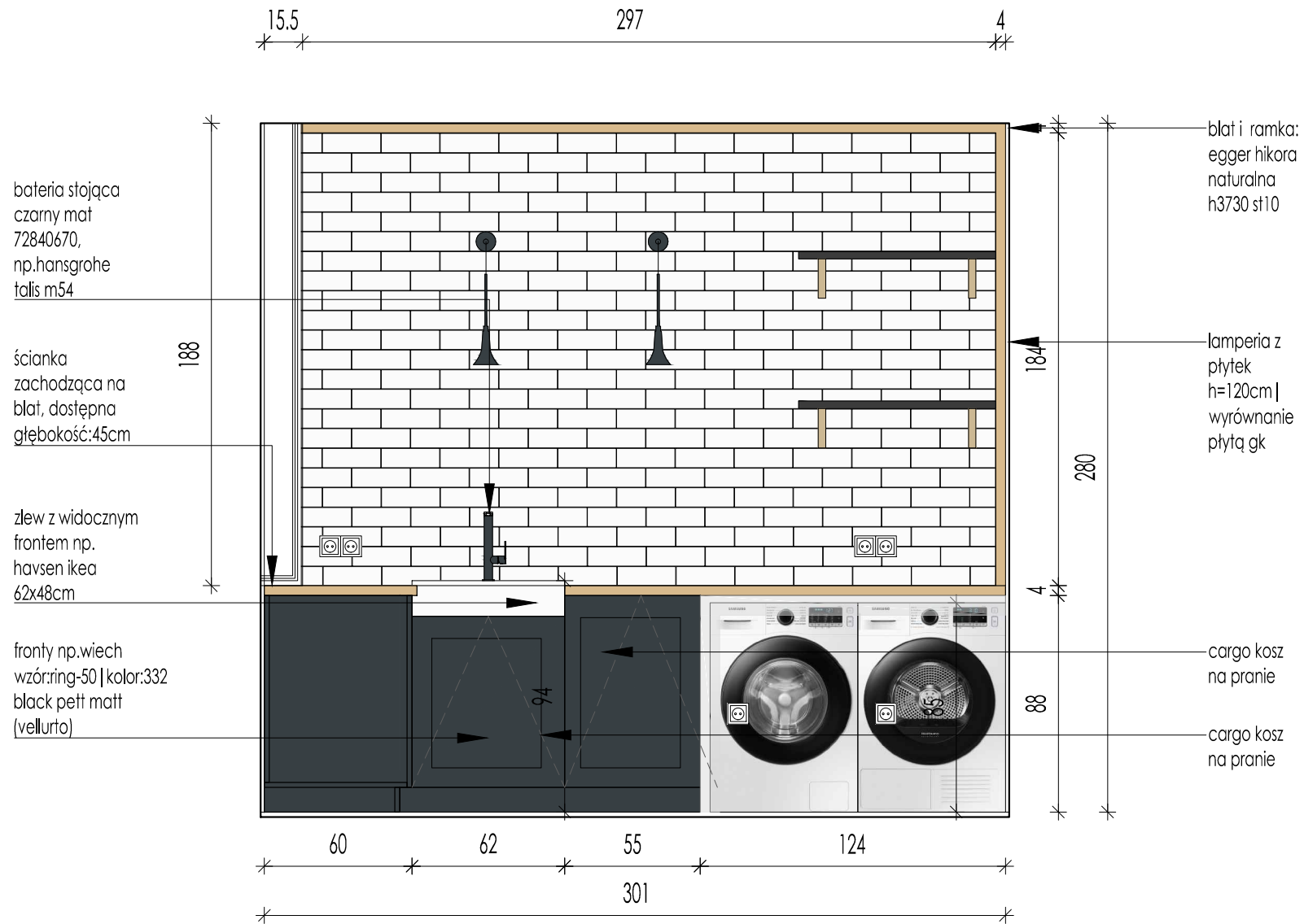
PRALNIA-WIDOK A-A
