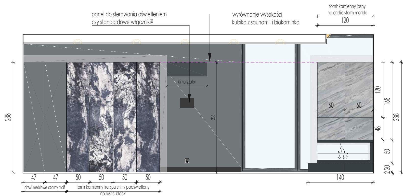
WIDOK B-B
