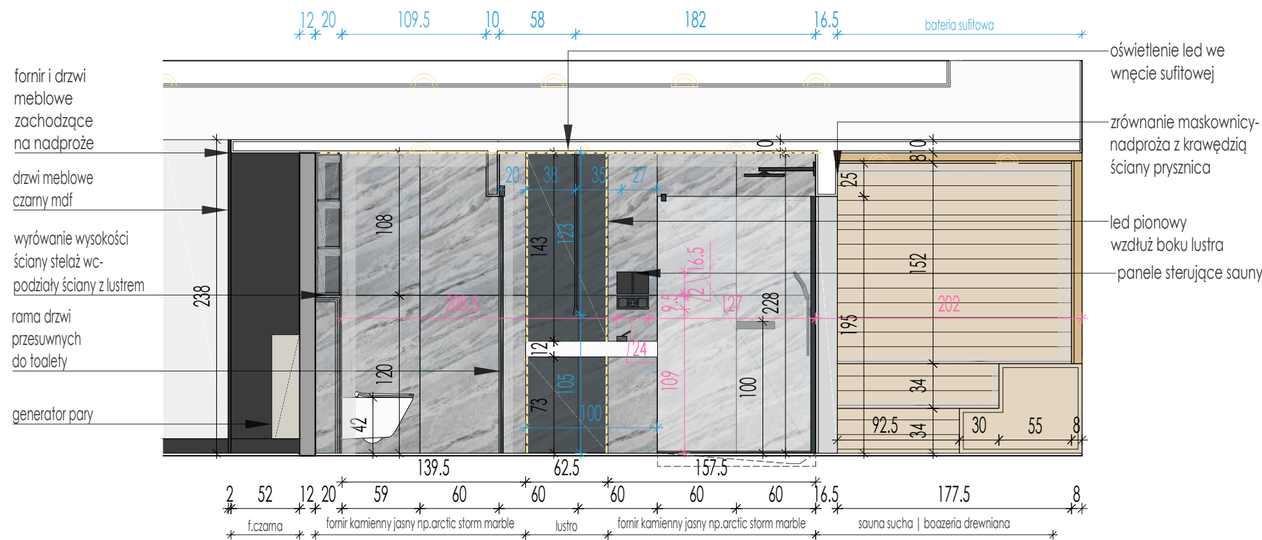
WIDOK F-F
