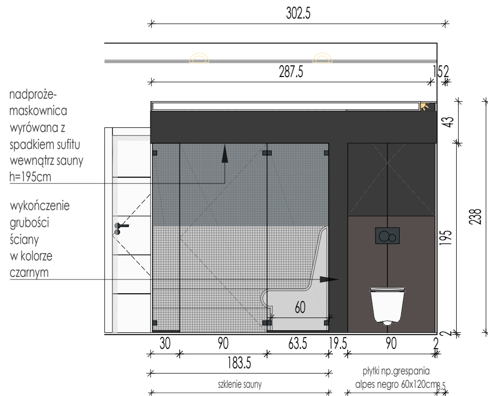
WIDOK G-G
