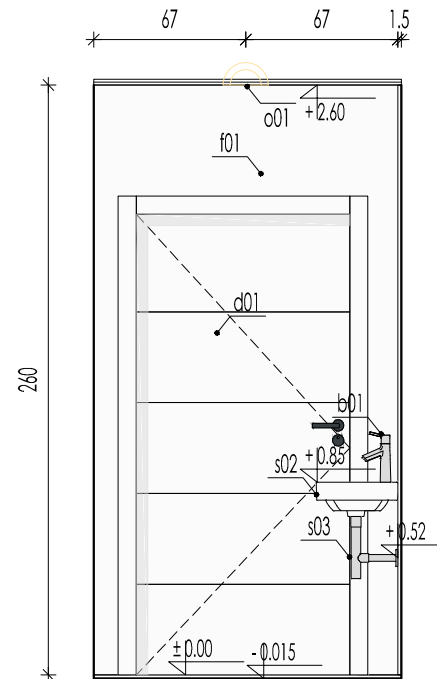
WIDOK D-D
