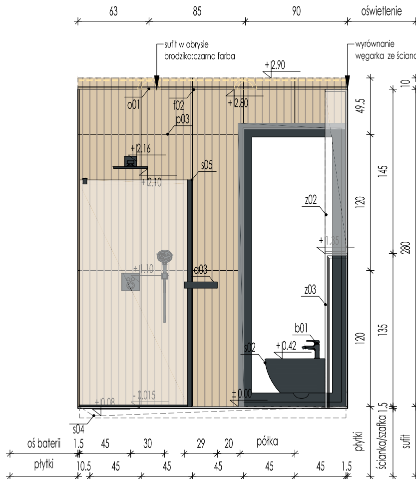
WIDOK B-B
