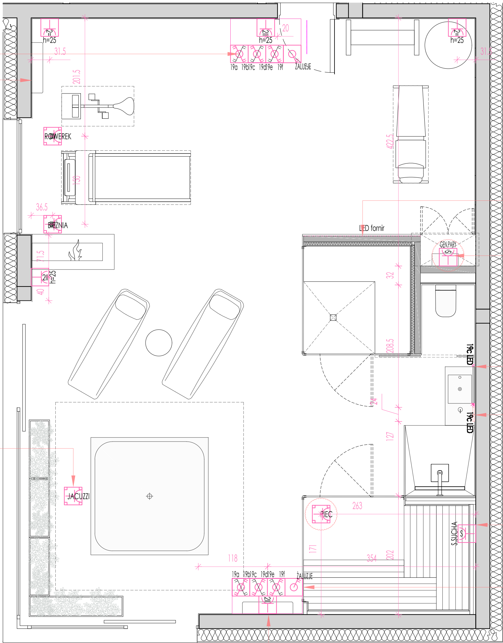
RZUT INSTALACJI ELEKTRYCZNEJ | ŚCIANY
