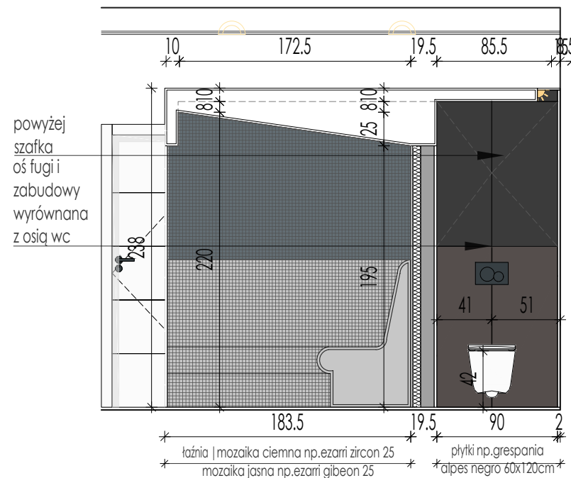
WIDOK H-H
