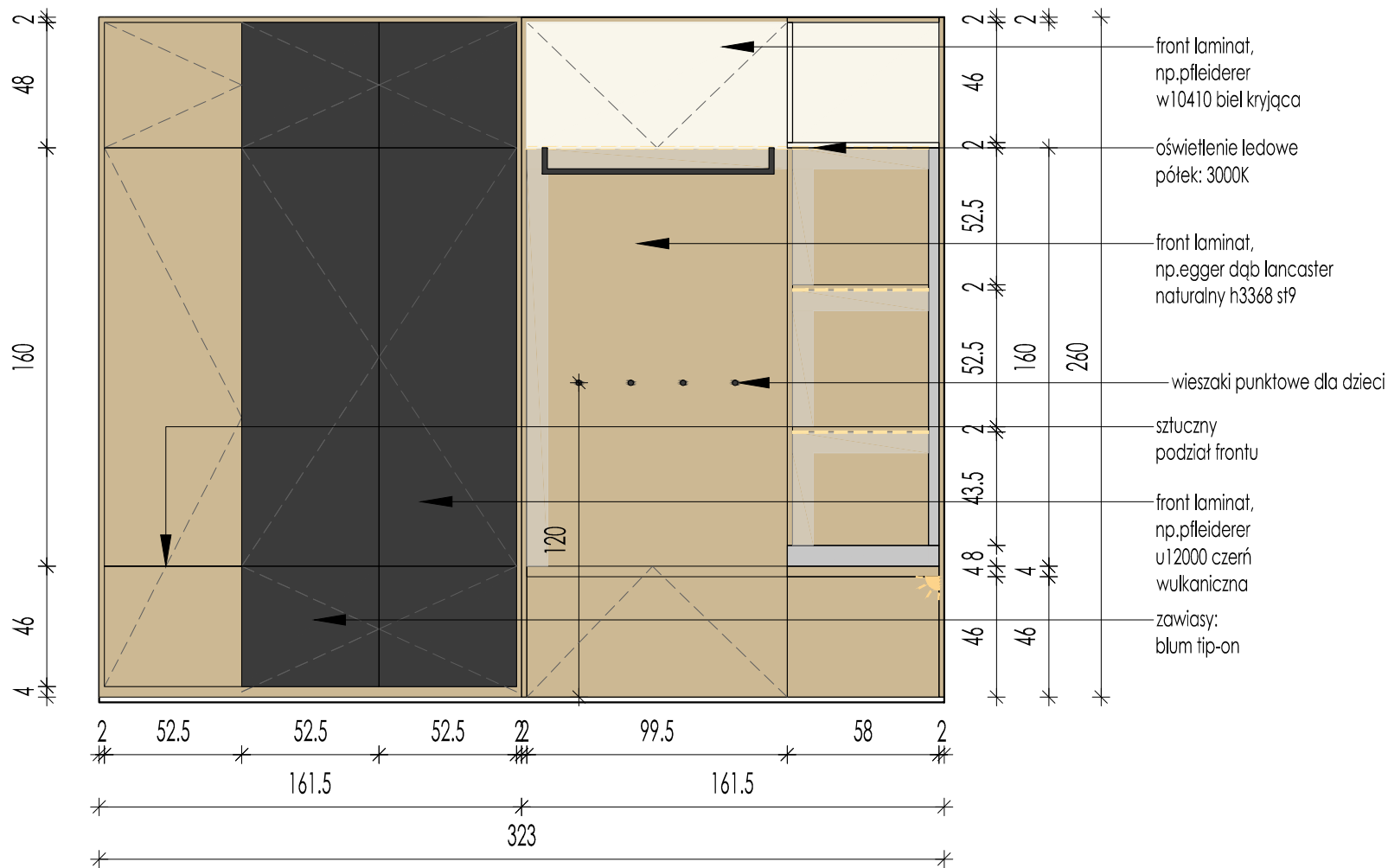
GARDEROBA PRZY HOLU-WIDOK B-B | ZAMKNIĘTA
