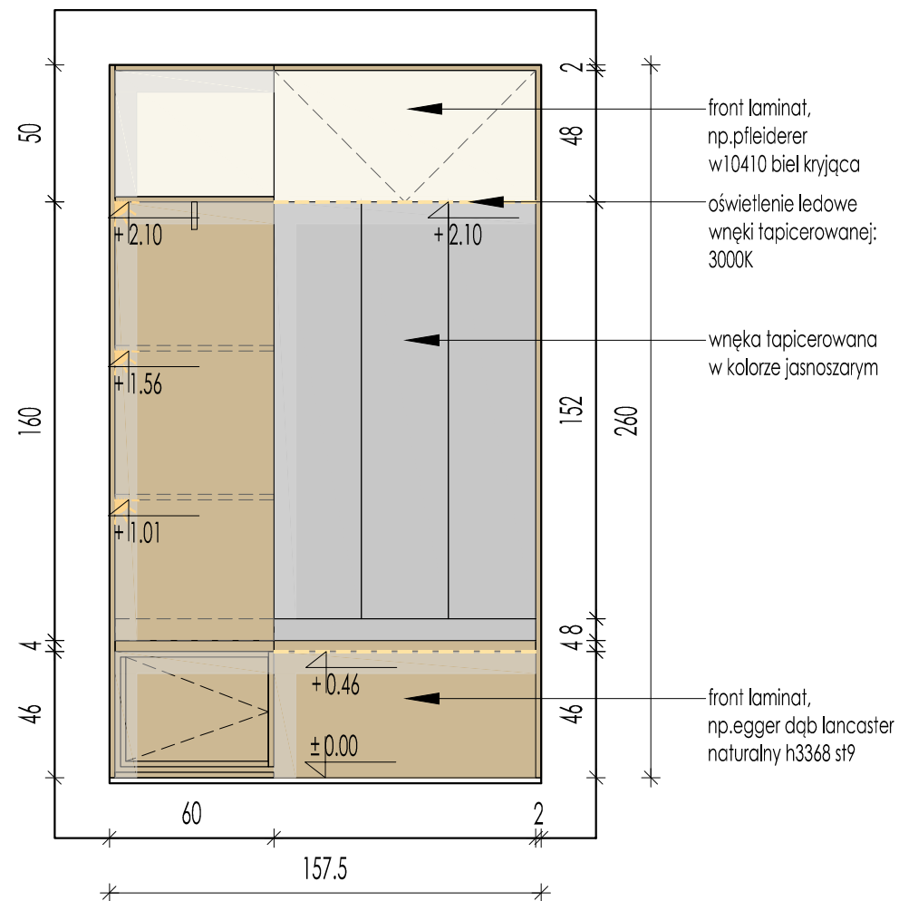
GARDEROBA PRZY HOLU-WIDOK A-A
