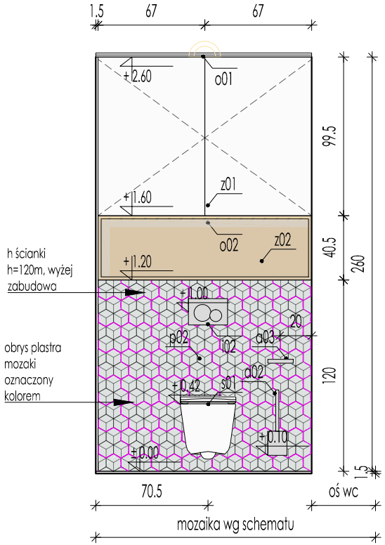
WIDOK B-B
