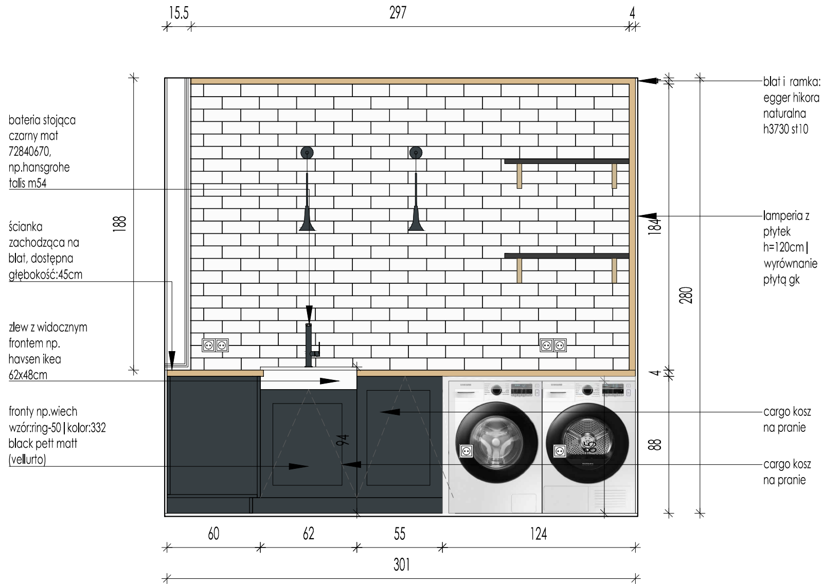
PRALNIA-WIDOK A-A
