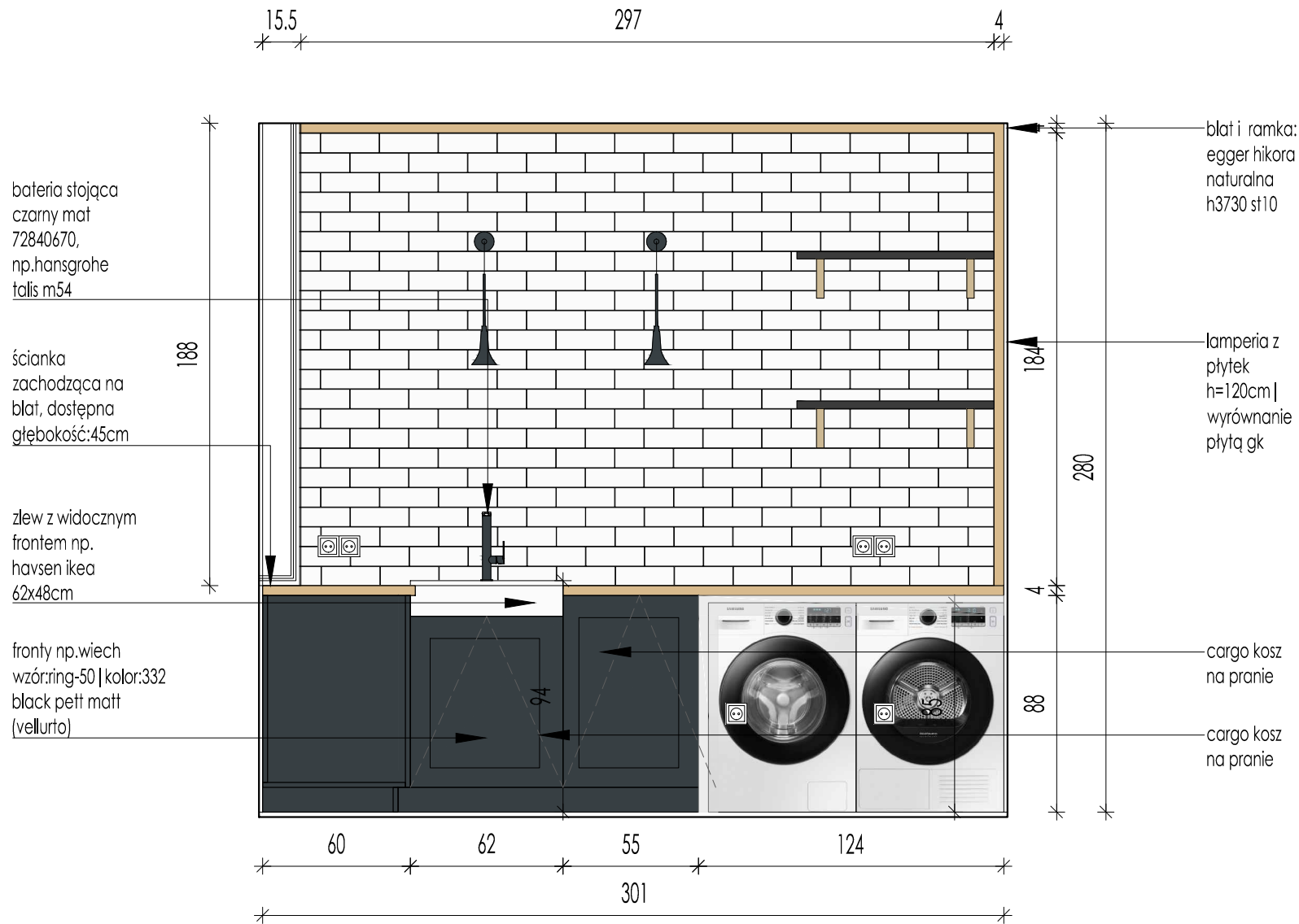
PRALNIA-WIDOK A-A
