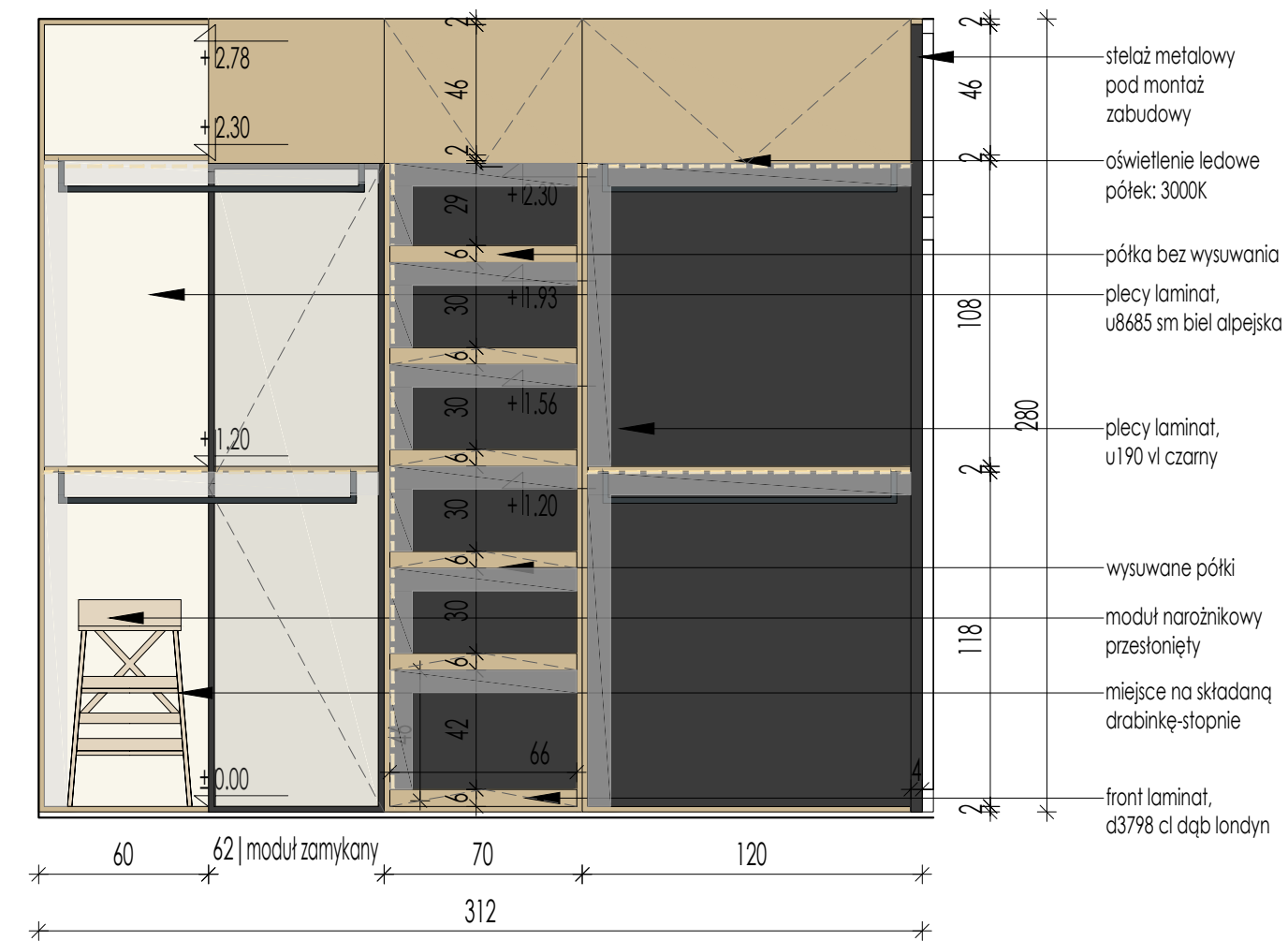
PIALNIA-WIDOK A-A
