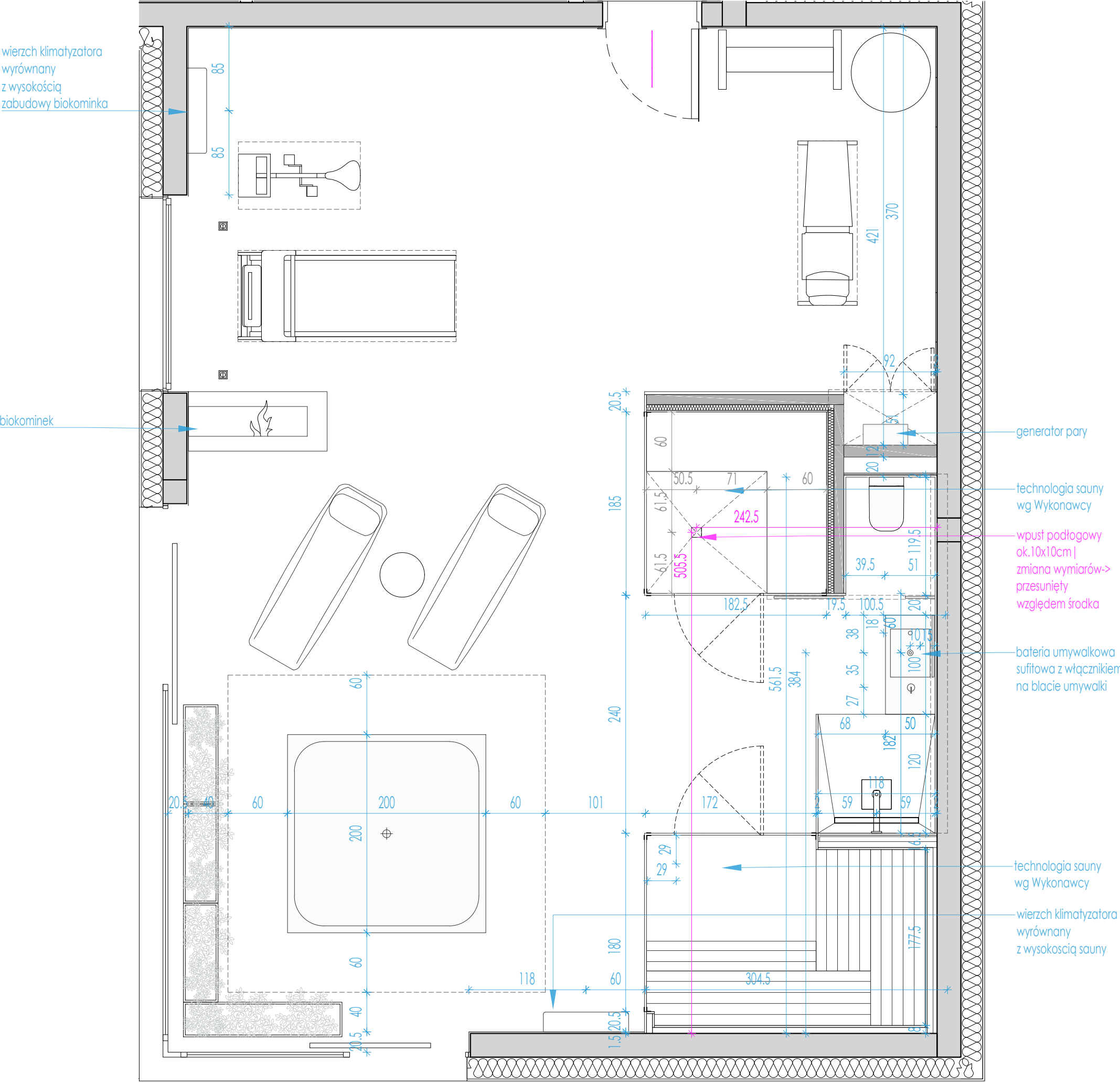
RZUT INSTALACJI SANITARNEJ
