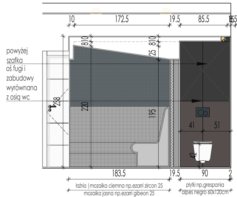
WIDOK H-H
