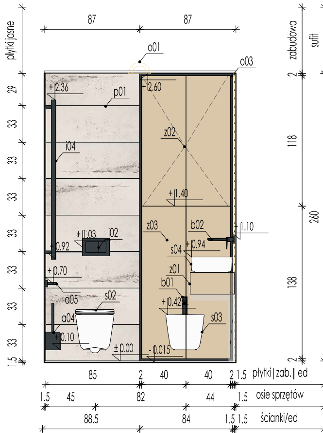
WIDOK D-D
